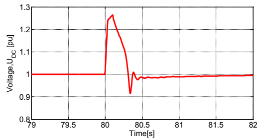
Fig. 12. DC-link voltage
