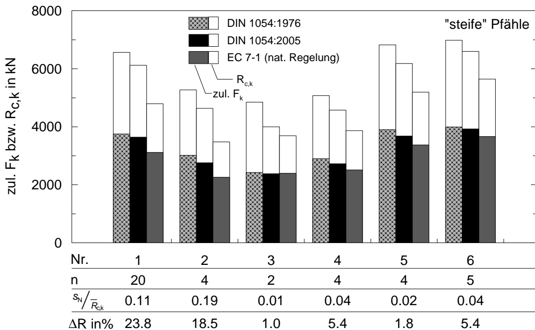
Bild 3 Vergleichende Pfahlwiderstände und zulässige Belastungen von Stahlrohrpfählen bei „steifen“ Pfählen und g_{G,Q} = 1,40 aus verschiedenen dynamischen Probelastungsergebnissen
