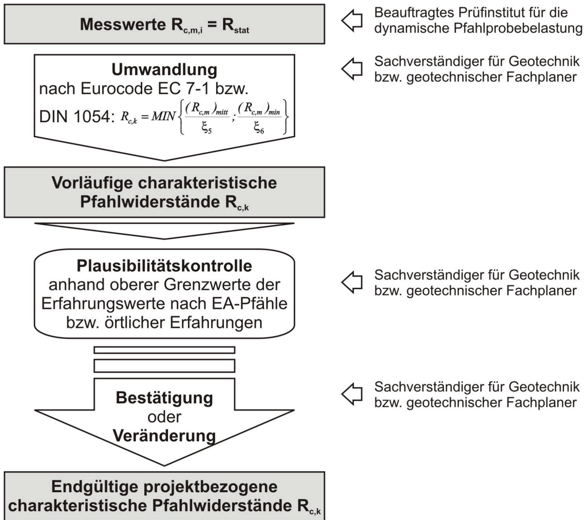
Bild 5 Bearbeitungsschritte nach EA-Pfähle und Ermittlung von charakteristischen Pfahlwiderständen aus den Messwerten bei dynamischen Pfahlprobelastungen
