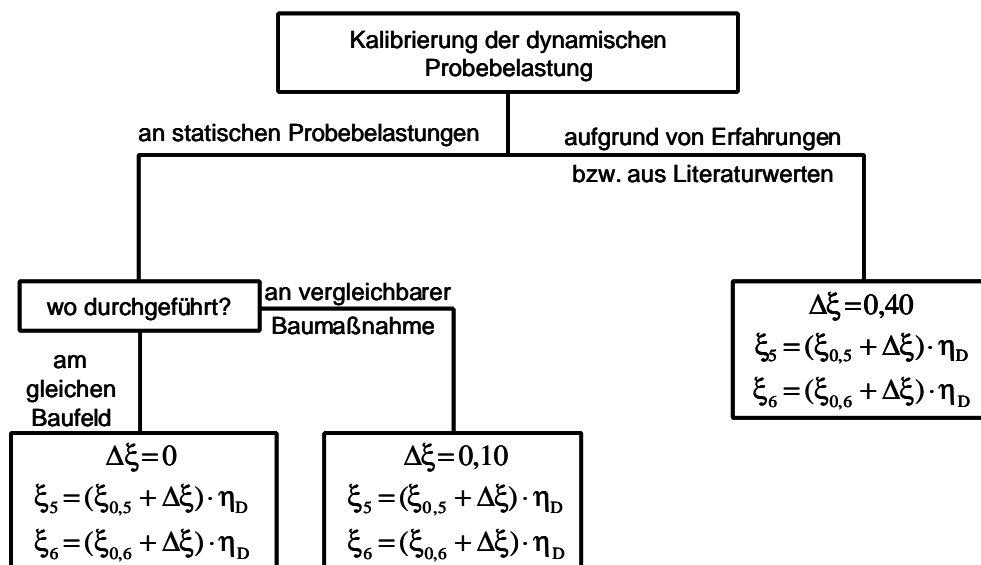
Bild 1 Diagramm zum Vorgehen bei der Ableitung der Streuungsfaktoren x nach Tabelle 3
