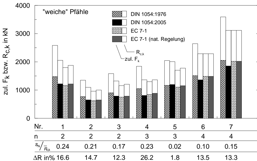
Bild 2 Vergleichende Pfahlwiderstände und zulässige Belastungen von Fertigrammpfählen (Stahlbeton) bei „weichen“ Pfählen und g_{G,Q} = 1,40 aus verschiedenen statischen Probelastungen
